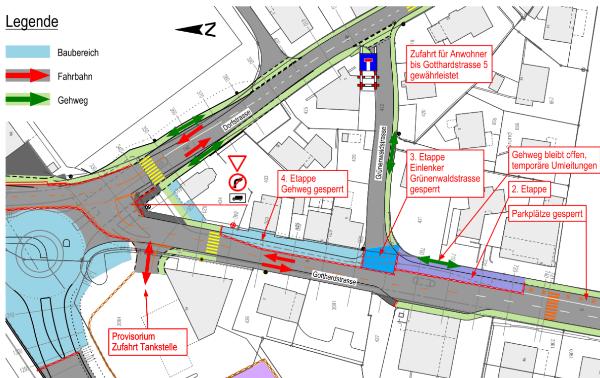
Übersichtsplan Verkehrs- und Fussgängerführung Ende Mai bis August 2025, Etappen 2 bis 4
